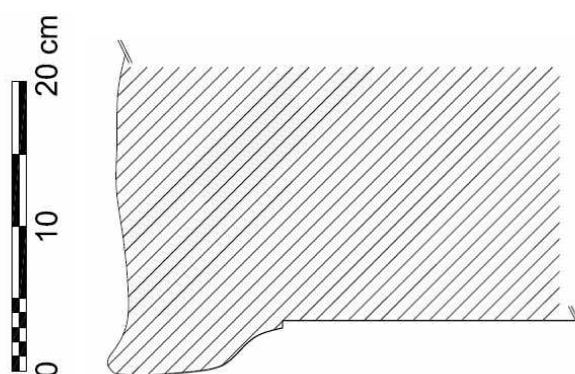
Obr. 6. Černěves, kostel sv. Prokopa, kresebné zobrazení profilu náběžního štítku profilace fragmentu ostění v ohradní zdi hřbitova. Autor: Táňa Nejezchlebová 2013.
