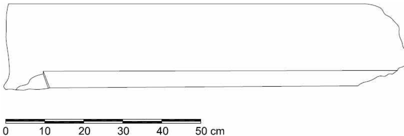
Obr. 4. Černěves, kostel sv. Prokopa, axonometrické zobrazení fragmentu ostění v ohradní zdi hřbitova. Autor: Táňa Nejezchlebová 2013.
