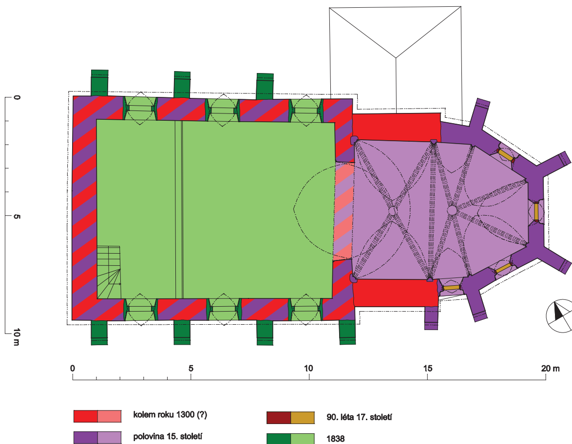
Obr. 5. Půdorysný řez vedený v úrovni okenních otvorů lodi a presbytáře. Zaměření a kresba: Tomáš Brož a Jaroslav Skopec, 2010. Vyhodnocení: Tomáš Brož a Jaroslav Skopec, 2016.
