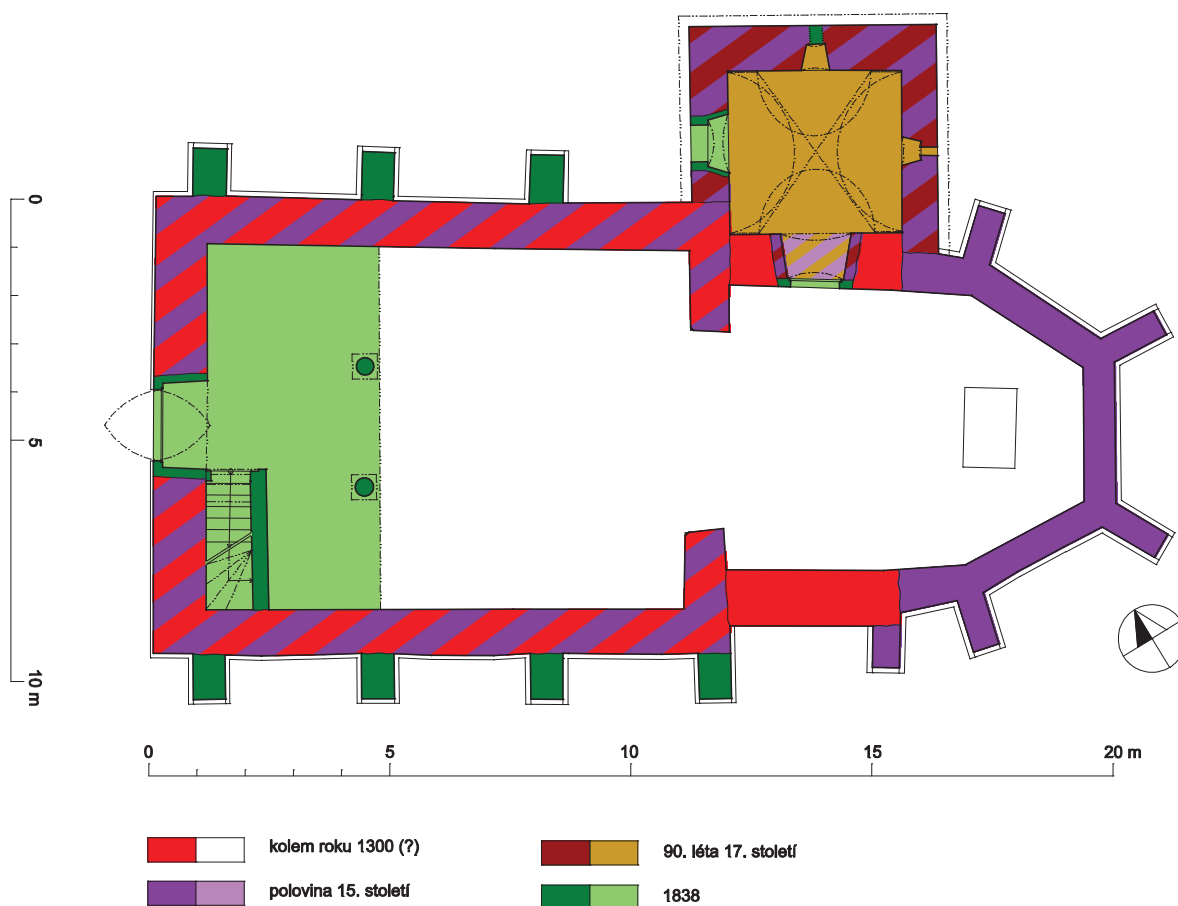
Obr. 4. Půdorysný řez vedený v úrovni vstupu s vyhodnocením stavebního vývoje. Zaměření a kresba: Tomáš Brož a Jaroslav Skopec, 2010. Vyhodnocení: Tomáš Brož a Jaroslav Skopec, 2016.
