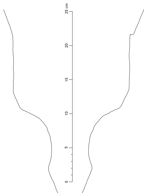
Obr. 10. Profil žebra klenby presbytáře. Zaměření a kresba: Jaroslav Skopec, 2010.
