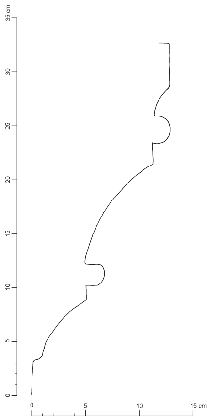
Obr. 12. Vertikální profil jižní konzole presbytáře. Zaměření a kresba: Jaroslav Skopec, 2010.
