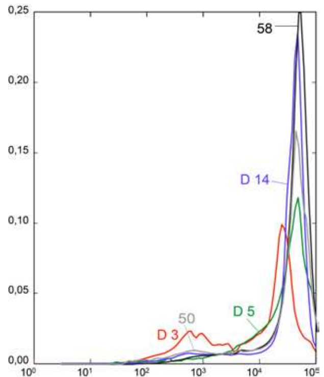
6) Grafy diferenciální distribuce velikosti pórů pro pískovce z různých staveb v Terezíně (D3, D5, D14) ve srovnání s grafy pro pískovce z lomu Spravedlnost v Děčíně (50) a z lomu Goldene Ranzen 3 (AZ sanace) v areálu Goldene Ranzen (58). Podrobnosti viz popiska obr. 5. Autor J. Adamovič.
