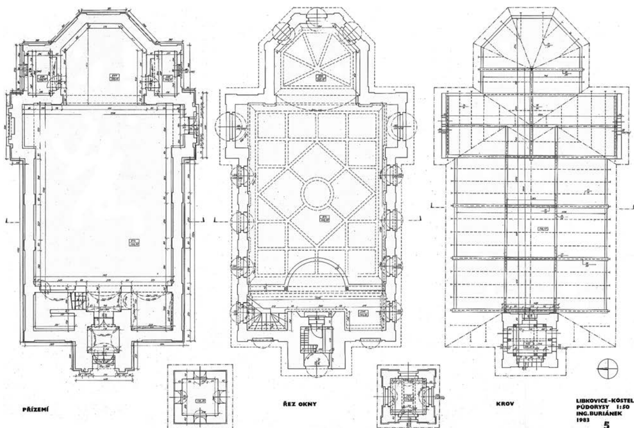
Obr 18. Kostel sv. Michaela, výkresová dokumentace pořizená před zničením kostela, půdorysy, Ing. Baláčková 1983, měřítko 1:50, archiv TO NPÚ ÚOP v Ústí nad Labem
