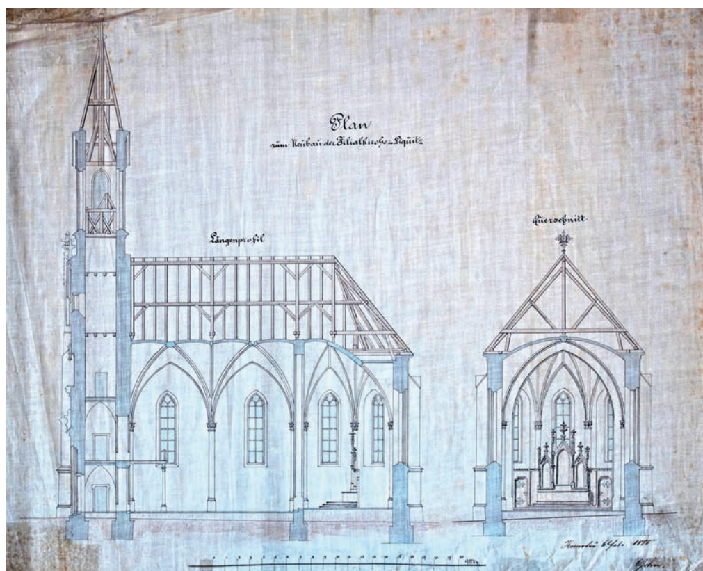
Obr 6. Výkresová dokumentace nerealizovaného návrhu nového filiálního kostela z roku 1885, autorem byl chomutovský architekt Carl John. Podélný a příčný pohled. Uloženo v SOA Litoměřice, fond ŘC Osek, inv. č. 13636, 13637, foto Kateřina Neumannová 2025, NPÚ ÚOP Ústí n. Labem.
