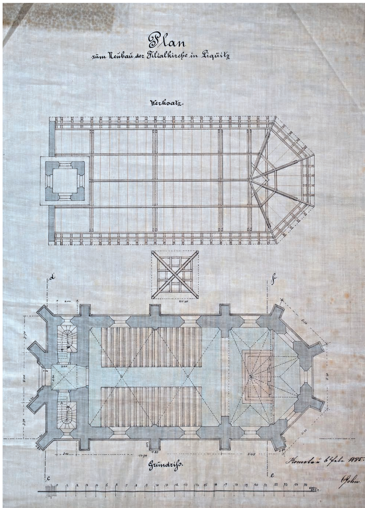
Obr 7. Výkresová dokumentace nerealizovaného návrhu nového filiálního kostela z roku 1885, autorem byl chomutovský architekt Carl John. Půdorys. Uloženo v SOA Litoměřice, fond ŘC Osek, inv. č. 13636, 13637, foto Kateřina Neumannová 2025, NPÚ ÚOP Ústí n. Labem
