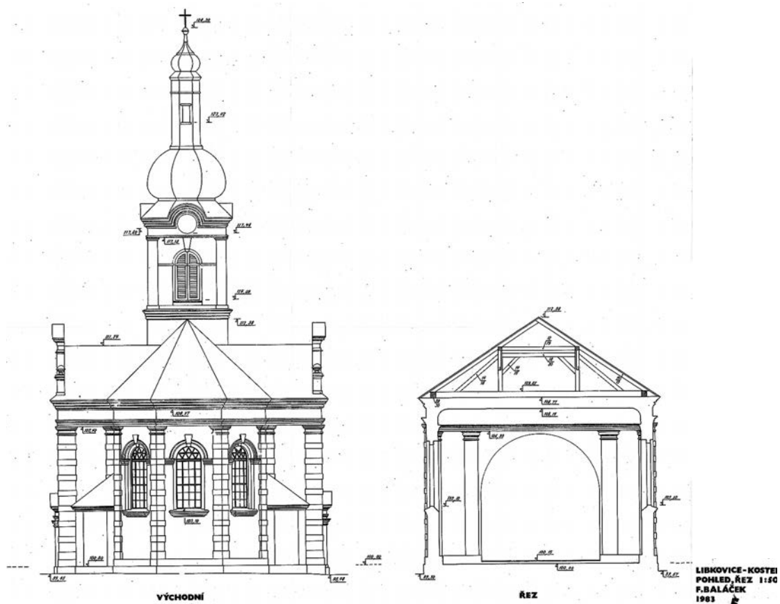
Obr 17. Kostel sv. Michaela, výkresová dokumentace pořizená před zničením kostela, východní pohled a řez, Ing. Baláčková 1983, měřítko 1:50, archiv TO NPÚ ÚOP v Ústí nad Labem
