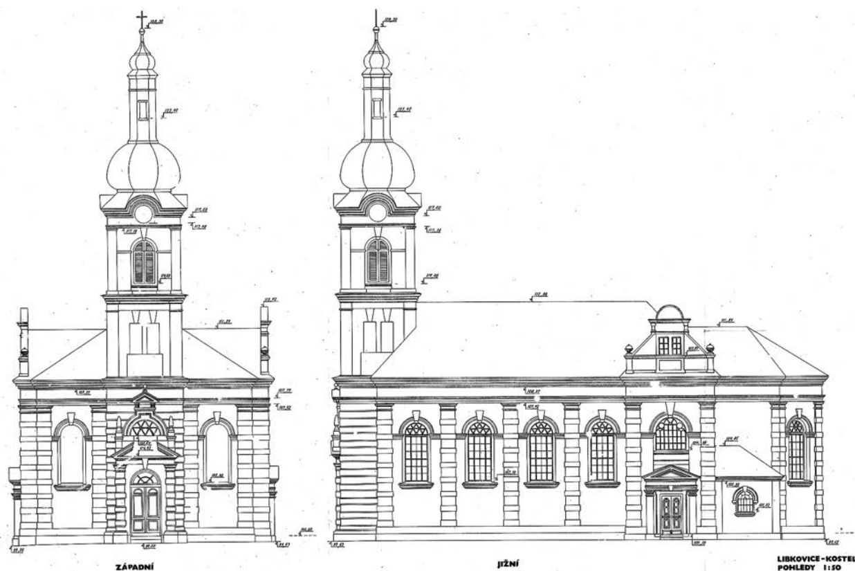
Obr 16. Kostel sv. Michaela, výkresová dokumentace pořizená před zničením kostela, západní a jižní pohled, Ing. Baláčková 1983, měřítko 1:50, archiv TO NPÚ ÚOP v Ústí nad Labem
